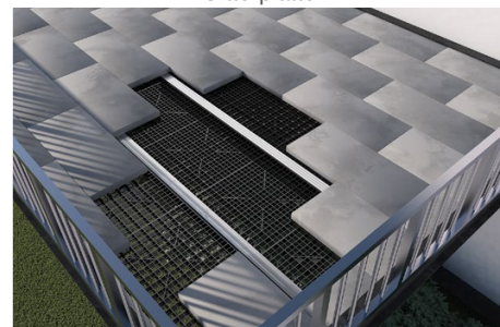
BERA Terrace Floor™ - Aufbau einer Terrasse/Balkon
