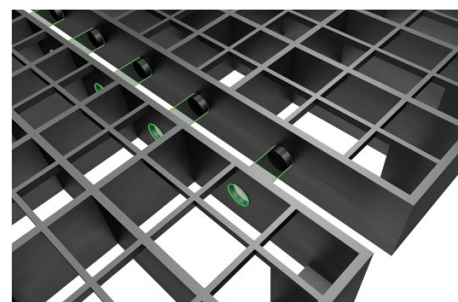
Integrierte seitliche Steck-Befestigung an Gitterplatte
