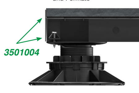
Fixierung der Gitterplatte (3501000) direkt auf Stelzlager
